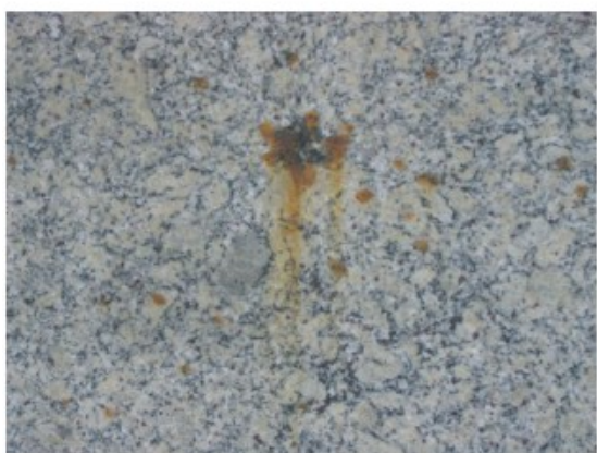
Foto 101 - Presença de mineral deletério (pirita), alterado por oxidação, manchando superfície polida de granito.
