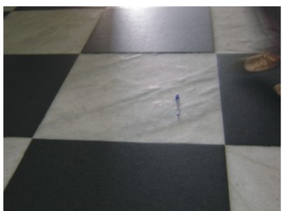
Foto 60 - Detalhe do piso da foto 62. Observar desgaste abrasivo mais elevado no mármore (branco).
