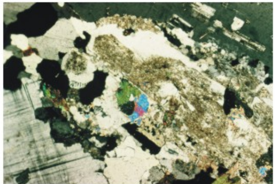
Foto 56 - Fotomicrografia do granito Cinza Mauá (São Paulo). Nicóis polarizados. Aumento de 20x.
