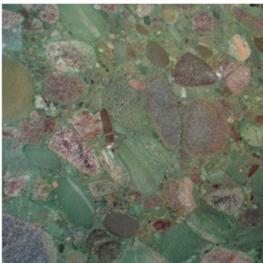
Foto 45 - Verde Caribe: metaconglomerado polimítico verde (Bahia).
