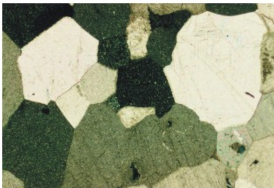
Foto 57 - Fotomicrografia de mármore branco (Espírito Santo). Nicóis polarizados. Aumento de 20x.
