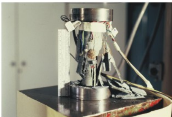
Foto 61 - Ensaio de resistência à compressão uniaxial (norma NBR 12767).
