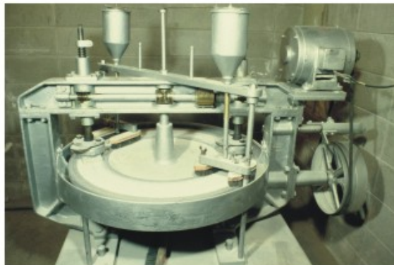
Foto 58 - Ensaio de resistência ao desgaste abrasivo. Teste Amsler (norma NBR-1242).
