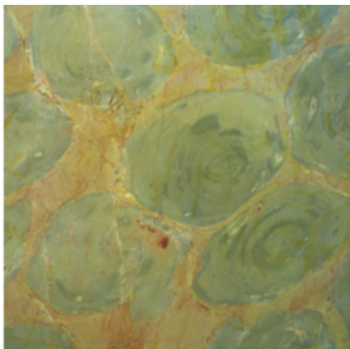
Foto 25 - Cappadocia: mármore fossilífero com estromatólitos (Paraná).
