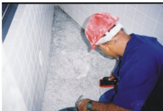
Foto 77 - Aplicação de rejuntamento cimentício industrializado. A argamassa é pressionada para dentro da junta, com desempenadeira de borracha.
