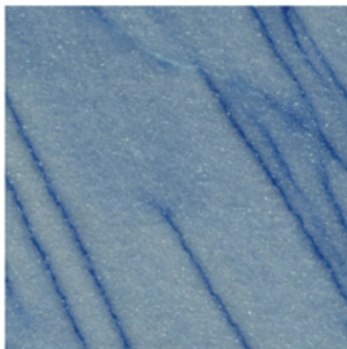
Foto 36 - Azul Boquira: quartzito maciço com dumortierita (Bahia).
