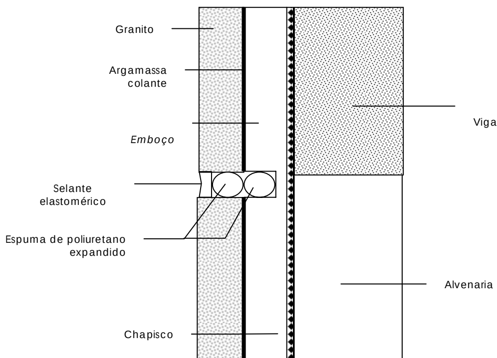
Fig. 4.3.1 – Exemplo de Junta de Movimentação (CARVALHO JR., 1999)
